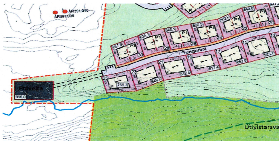
Mynd 1 Staðsetning fráveitumannvirkis við enda Tungurima, Reykholti, Bláskógabyggð - Heimild deiliskipulagsuppráttur
