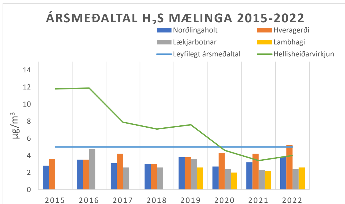
Mynd 21. Samanburður ármeðaltals H_2S mælinga milli ára
